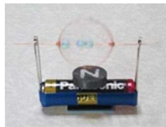
【コイルモーターに電気を通すとコイルが勢いよく回り出します】
